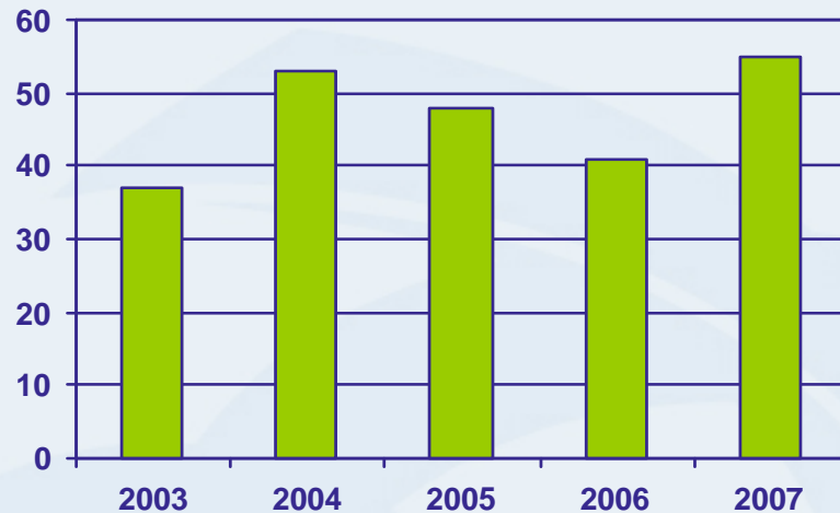
IPv6 - Prefixes
